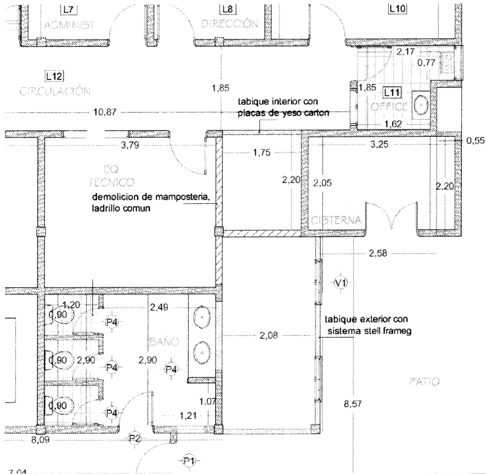
Planta CVE y CVI nuevos y a demoler
