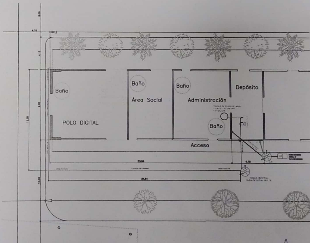
Plano instalación sanitaria Esc 1:200
