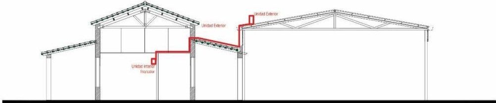
CORTE TRANSVERSAL TRAZADO DE AIRE
